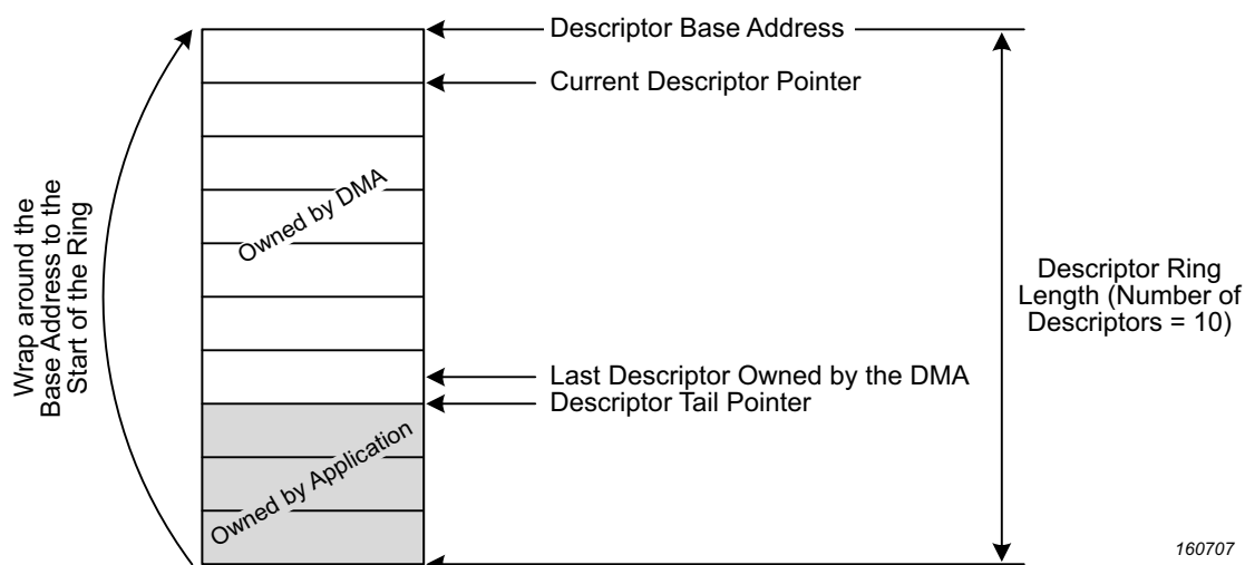
Fig 166. Descriptor ring
